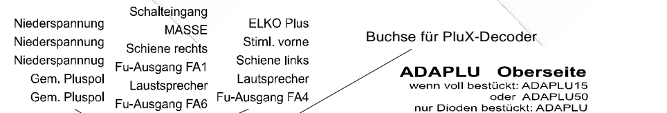
ADAPLU - ohne Niederspannungsquelle ADAPLU15 oder ADAPLU50 - Niederspannung 1,5 bzw. 5V
